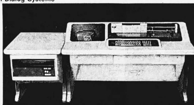
RUF-Computer mit Plattenspeichern, mit Floppy-Disketten, mit oder ohne Magnetknoten
