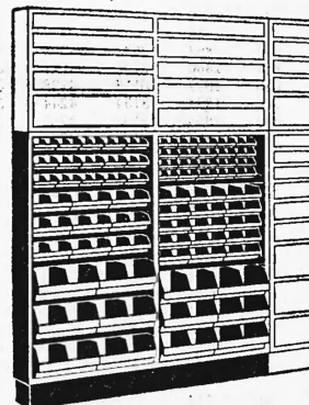
AUFBAUREGAL in Einzelelementen SICHTLAGERKASTEN in 5 Größen
