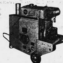
Appareil mobile de CHAUFFAGE D'AIR «HERMAN NELSON»
