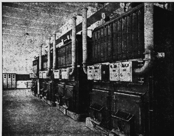
Großheizwerk mit 8 ØERTLI-Zwillingsbrennern an vier SULZER-Taschenkesseln
