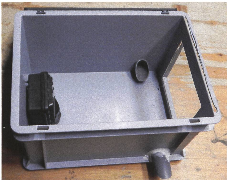
Abbildung 1: Prototyp der MiniMammalCamBox. Innenansicht der ersten Variante der MiniMammalCamBox aus einer Rako-Box und einer speziell auf Kleinsäuger ausgerichteten Fotofalle, mit gegenüberliegendem, grossem Fenster aus Glas und seitlichen Eingängen aus PVC-Röhren. Dieser Prototyp wurde im Laufe der letzten Jahre optimiert (z. B. ohne Glas und Anbringung der Fotofalle an der langen Seite der Kiste), siehe Abbildung 3. Foto: Lorenzo Vinciguerra.
