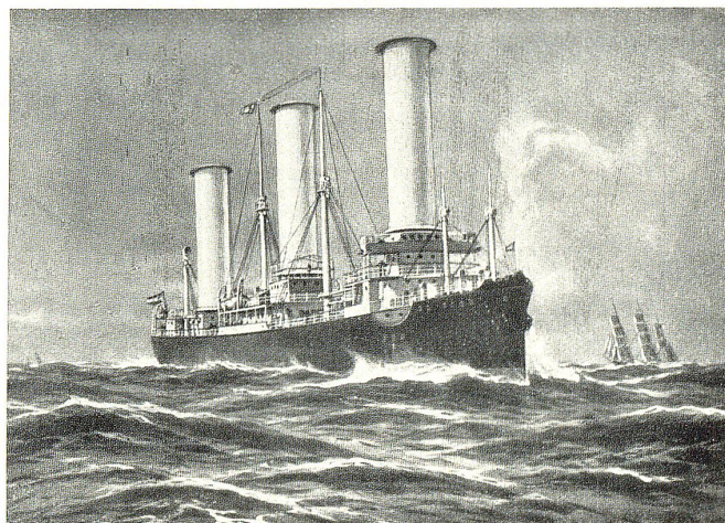
Neues 3000-Tonnen-Rotorschiff, erbaut von der Seetransport-Abteilung der deutschen Reichsmarine (aus Flettner: Mein Weg zum Rotor).
