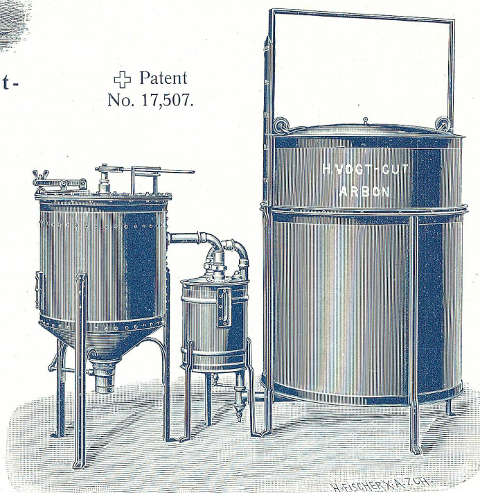
Käserei-Feuerungs-Anlagen
