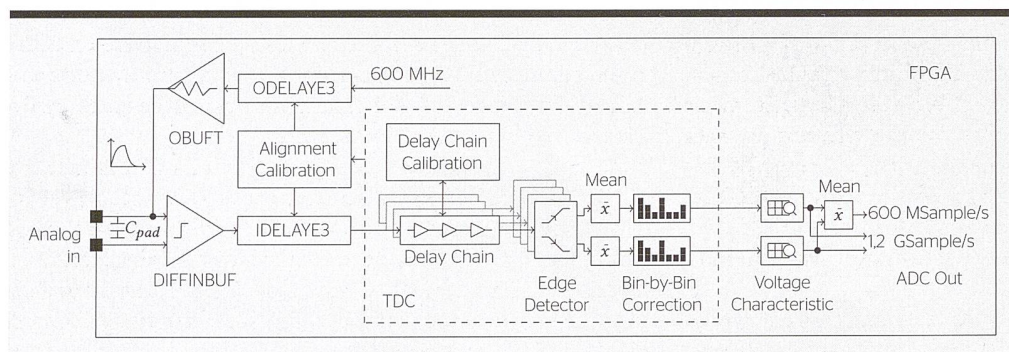
Bild 2 Architektur des neuartigen FPGA-basierten ADCs.
