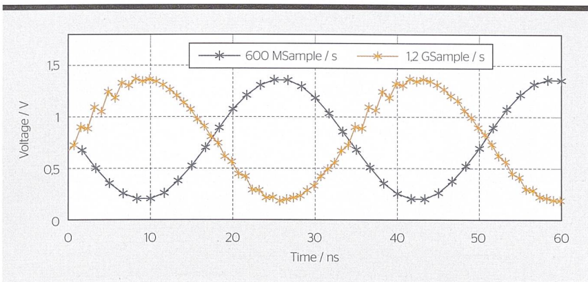
Bild 3 Messung eines 30-MHz-Sinus.
