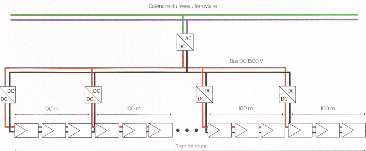
Figure 3 Architecture d'une installation PV linéaire en emprise ferroviaire installée en bordure de voie ou entre les rails (solution Sun-Ways).
