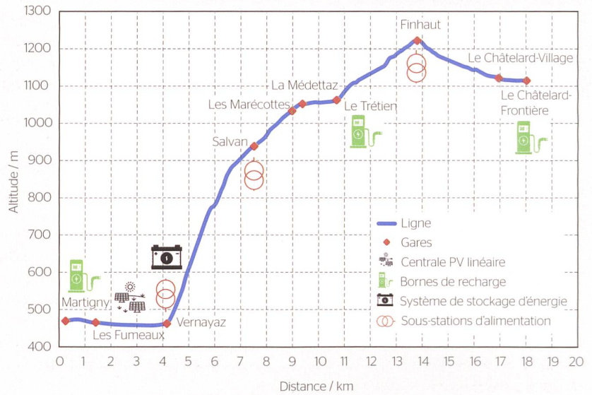
Figure 4 Profil de la ligne ferroviaire Martigny - Le Châtelard et position des microgrids ferroviaires pour la recharge des véhicules électriques à proximité des gares.
