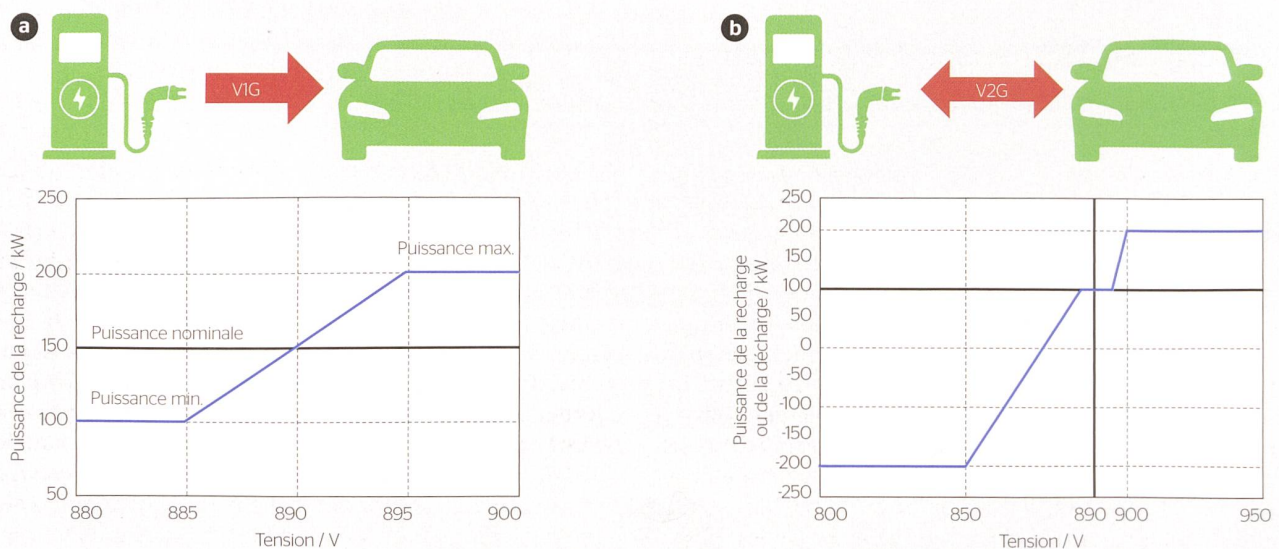
Figure 5 Paramétrage du système de gestion de l'énergie basé sur une fonction « droop control » : a) pour la recharge intelligente (V1G), et b) pour la recharge bidirectionnelle (V2G).
