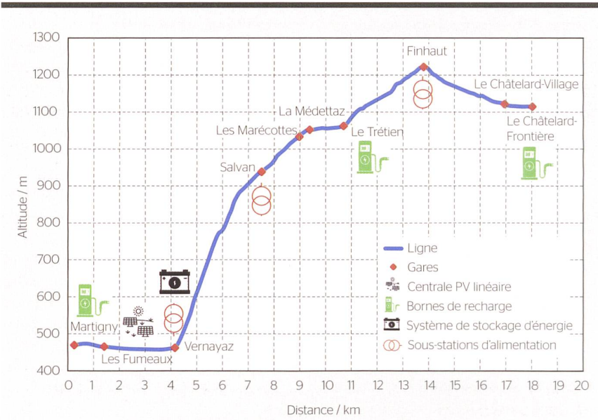
Figure 4 Profil de la ligne ferroviaire Martigny - Le Châtelard et position des microgrids ferroviaires pour la recharge des véhicules électriques à proximité des gares.
