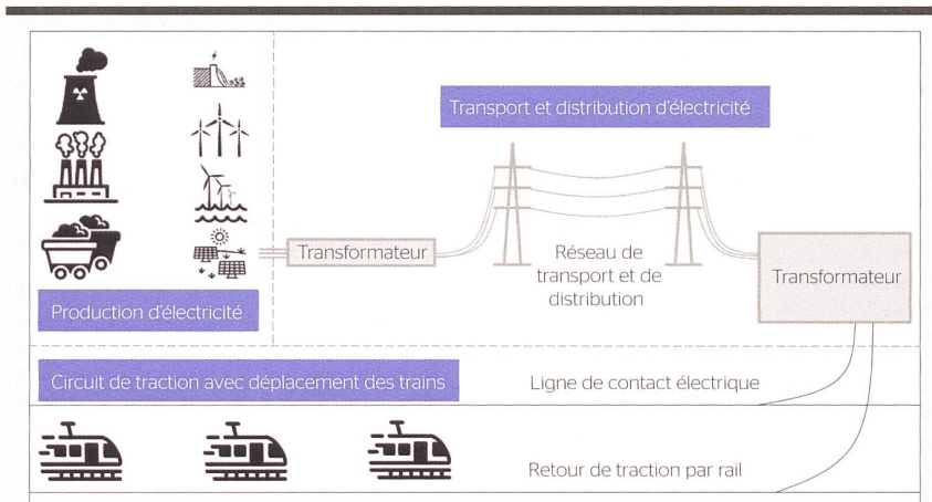
Figure 1 Schéma de l'infrastructure électrique ferroviaire.
