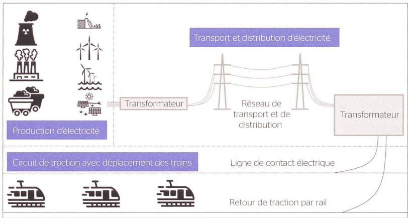
Figure 1 Schéma de l'infrastructure électrique ferroviaire.
