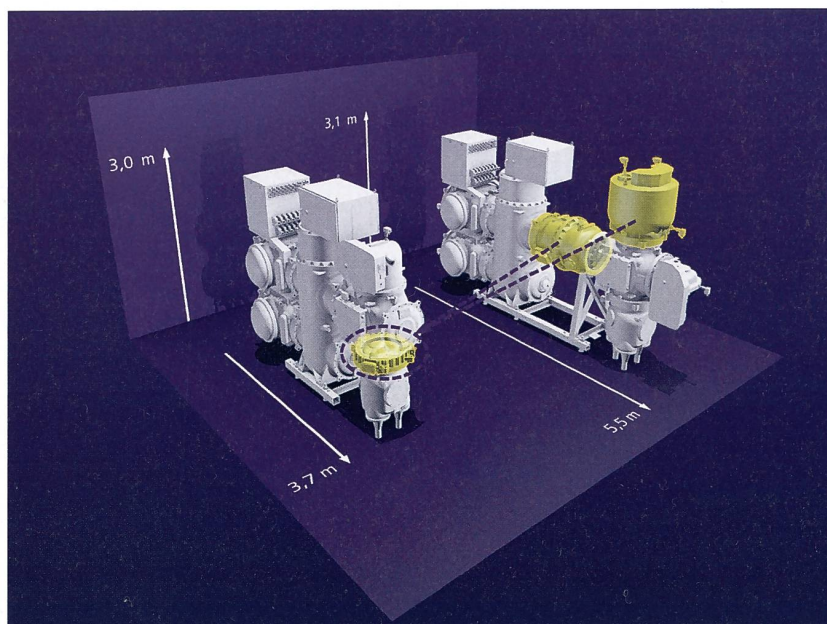
Bild 1 145-kV-BlueGIS: 1500 kg Materialersparnis und 30 % Feldlängenreduktion dank LPIT im beispielhaften Feldaufbau.
