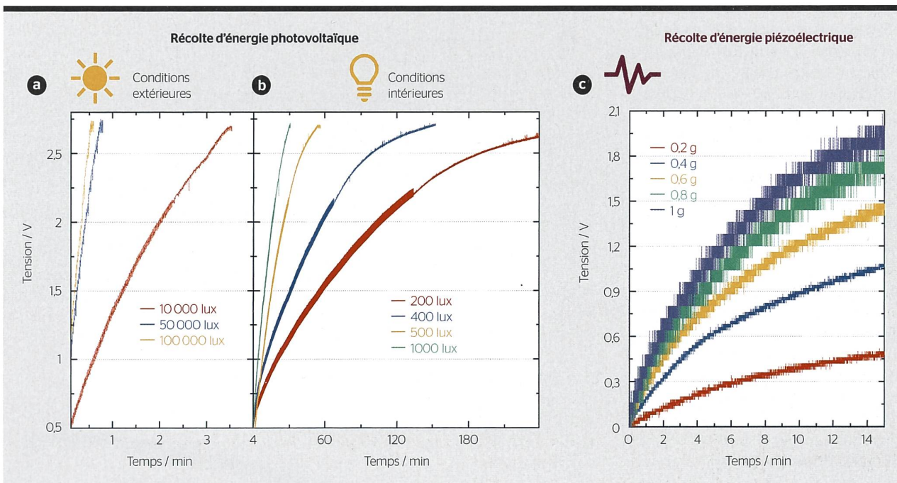
Figure 3 Caractéristiques de charge d'un supercondensateur : a) de 200 mF avec une cellule solaire dans des conditions de lumière extérieure intense et b) dans des conditions de faible luminosité intérieure, et c) de 50 mF avec trois dispositifs piézoélectriques soumis à des vibrations à une fréquence cible pour les applications automobiles.
