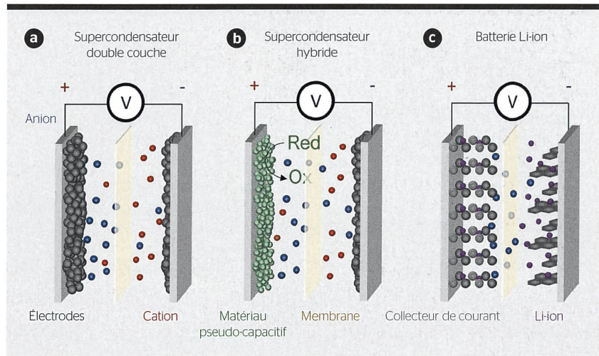
Figure 1 Les différents dispositifs de stockage d'énergie capacitive : a) le supercondensateur double couche, b) le supercondensateur hybride, et c) la batterie Li-ion.
