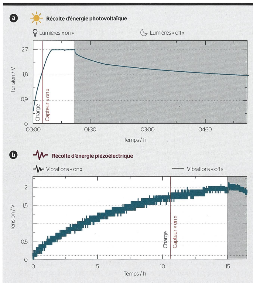
Figure 4 Caractéristiques des supercondensateurs pendant et après la charge ainsi qu'avant et pendant le fonctionnement continu d'un capteur enregistrant et transmettant des données toutes les 5 min : a) avec un dispositif de récolte d'énergie photovoltaïque et b) avec un système de récolte d'énergie piézoélectrique.
