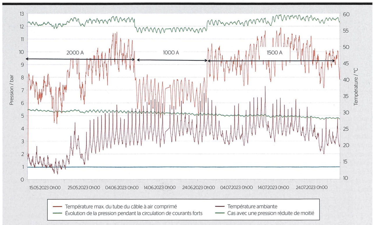
Figure 3 Au cours de l'année d'exploitation continue, le câble à air comprimé de l'installation de démonstration a été soumis pendant plusieurs semaines à des tests avec des courants permanents de différentes intensités (1000 A, 1500 A et 2000 A). La température du tube du câble à air comprimé n'a jamais dépassé 57°C et est donc toujours restée en dessous de la valeur limite de 65°C.
