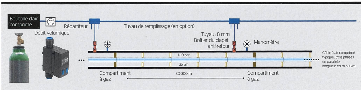
Figure 4 Selon les indications du fabricant, les câbles à air comprimé ne devraient présenter aucune perte de pression pendant leur durée de vie de 40 ans. Il peut toutefois arriver qu'il faille rajouter de l'air comprimé après des dommages ou des travaux de révision: les lignes à air comprimé sont donc équipées d'une alimentation en gaz à partir de bouteilles d'air comprimé.
