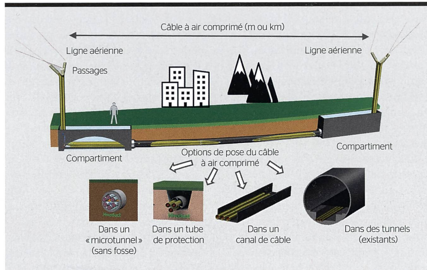
Figure 1 Représentation schématique d'une ligne à haute tension dont un tronçon est constitué d'un câble souterrain à air comprimé, avec quatre options différentes pour la pose du câble.
