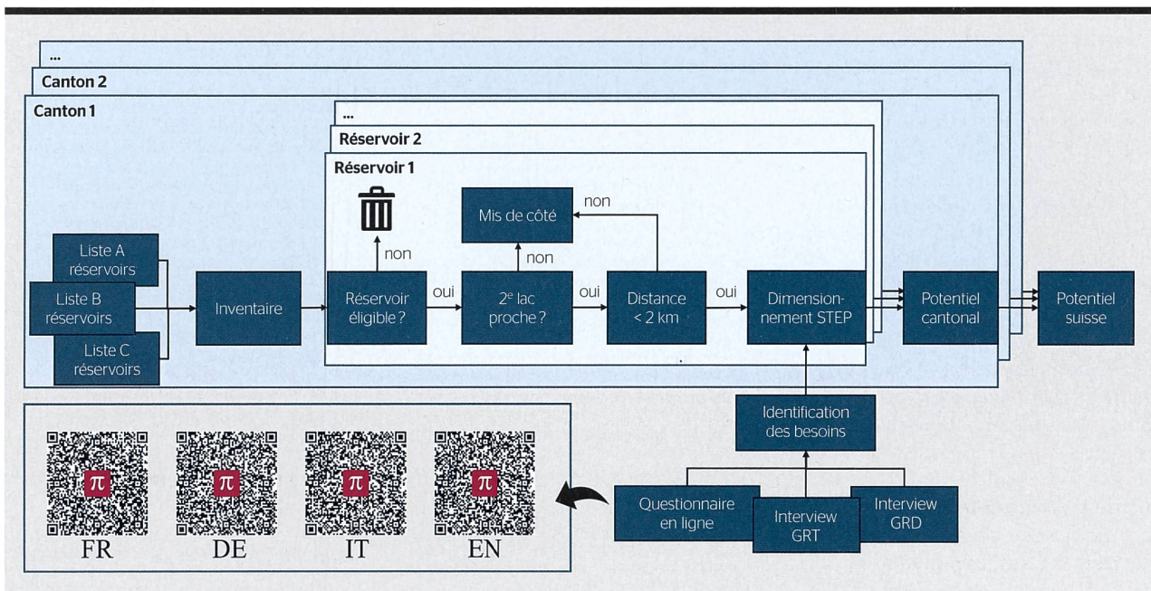
Figure 4 Méthode de sélection des sites de pompage-turbinage afin d'estimer le potentiel technique et liens vers les questionnaires en ligne.
