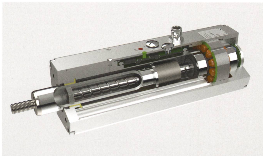
Bild 1 Blick ins Innere des Elektrozyinders: Der Servomotor (rechts) treibt eine Spindel (links) an, welche die lineare Hin-und-her-Bewegung hervorruft. Mittig über der Spindel ist die Bedienkonsole mit dem Potentiometer angebracht, direkt darunter die Servoregler-Elektronik.
