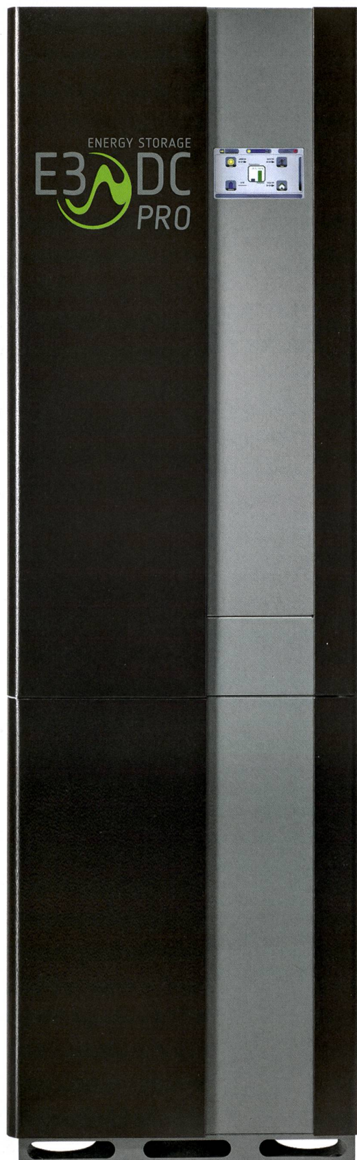
Centrale domestique E3/DC S10E Pro Compact, une alimentation de secours triphasée.
