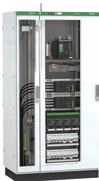
PrismaSeT P Active mit eingebautem ComPact NSX und HeatTag.
