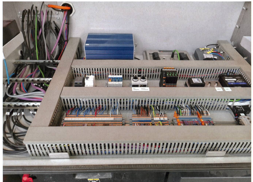
Eine Sicherheitssteuerung mit zwei unabhängigen Prozessoren und diversen Sensoren für Lage, Gewicht und Druck garantieren einen sicheren Betrieb.
