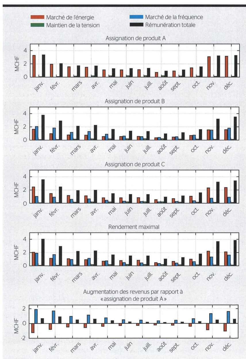
Figure 5 Résultats d'assignations de produit en tenant compte des trois paramètres suivants : réglage secondaire, prix du marché Swissmix et priorisation des sources de production décentralisée.
