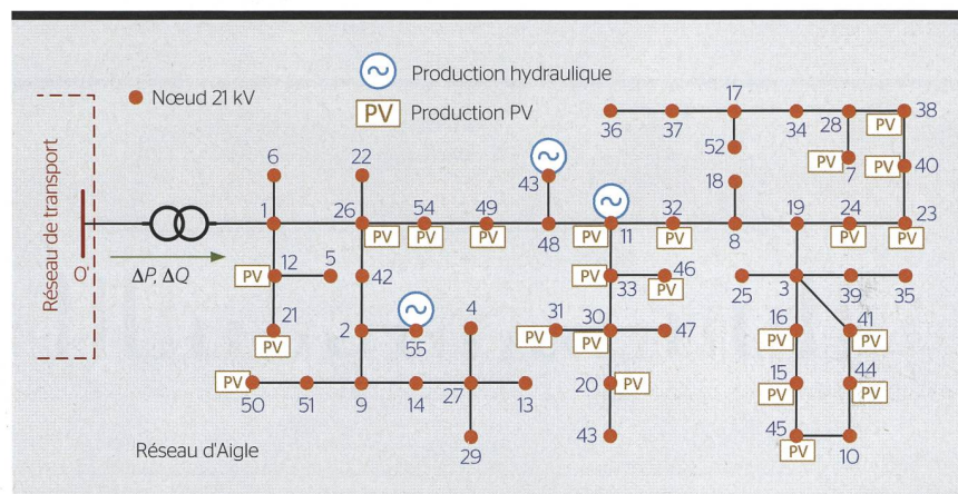
Figure 2 Schéma électrique du réseau d'Aigle.
