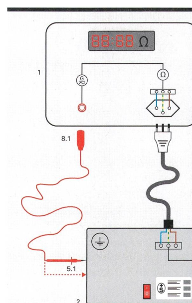
Figure 3 Schéma D.4.3 pour la mesure de la résistance du conducteur de protection.
