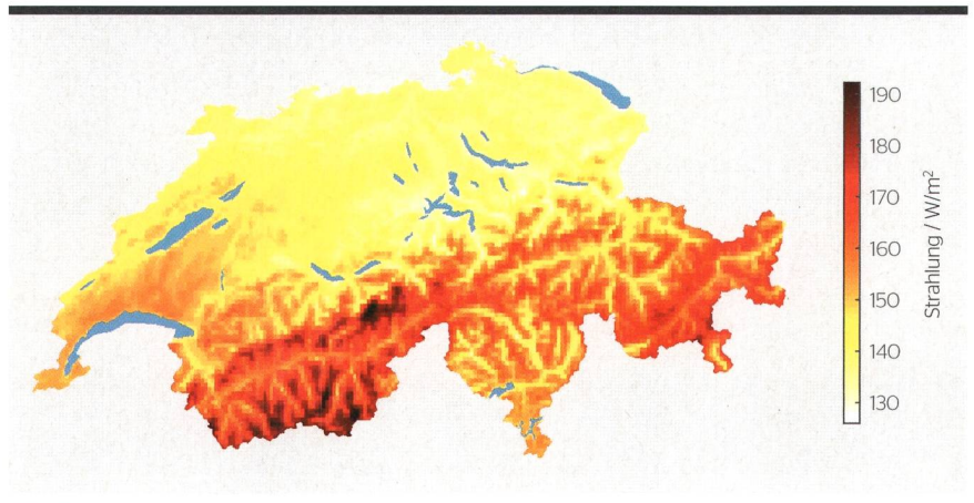
Bild 2 Langjähriges Mittel der Sonneneinstrahlung in der Schweiz.
