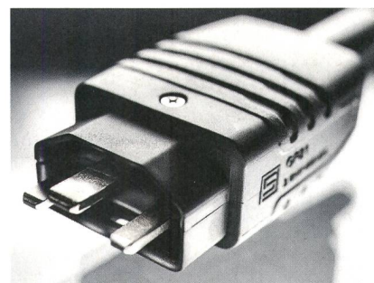
Stecker GP21 gemäss IEC TS 62735-1.
