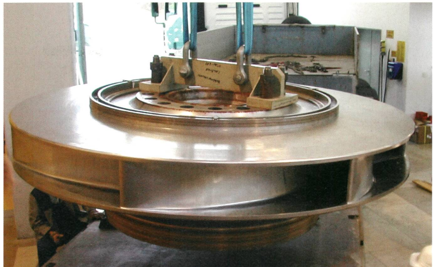
Bild 1 Laufrad einer Francis-Pumpturbine, Aussendurchmesser 3,0 m, Betriebsdrehzahl 8,35 s -1 , Durchfluss ≤32 m 3 /s.
