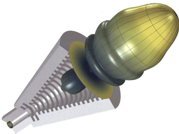
Abbildung des Fernfelds einer gewellten Rundhornantenne.
