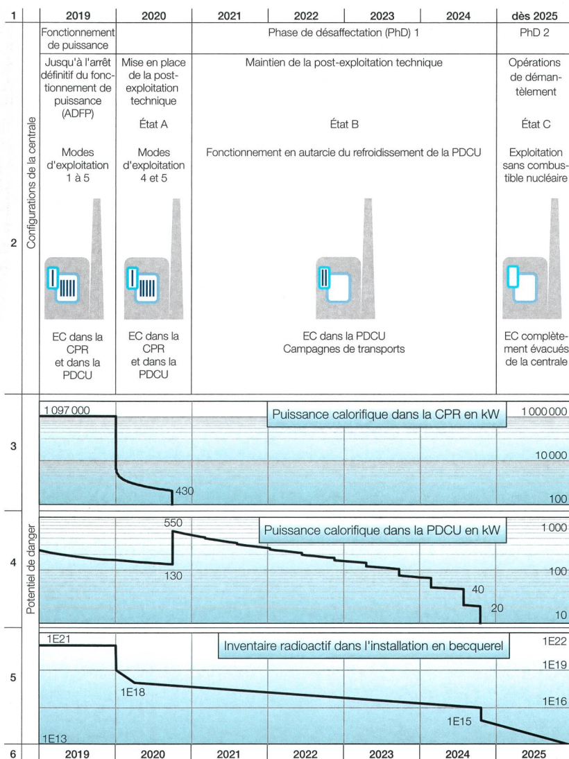
Figure 3 Potentiel de risque. À l'issue de l'ADFP, la puissance calorifique de la cuve sous pression du réacteur (CPR) chute à environ un millièème en l'espace de trois mois, par comparaison avec le fonctionnement de puissance. Le déplacement des éléments combustibles (EC) de la cuve sous pression du réacteur dans la piscine de désactivation du combustible usagé (PDCU) permet de réduire la puissance calorifique du CPR à pratiquement zéro, alors qu'elle augmente naturellement, dans un premier temps, dans la piscine de désactivation. La puissance calorifique continue de diminuer à chaque transport vers le centre de stockage intermédiaire de Würenlingen. Parallèlement, le potentiel de risque de l'installation exprimé en termes d'inventaire radioactif diminue. Si les combustibles nucléaires sont entièrement évacués de l'installation d'ici à la fin de l'année 2024, l'inventaire radioactif aura chuté à moins d'un millionième par comparaison avec le fonctionnement de puissance.
