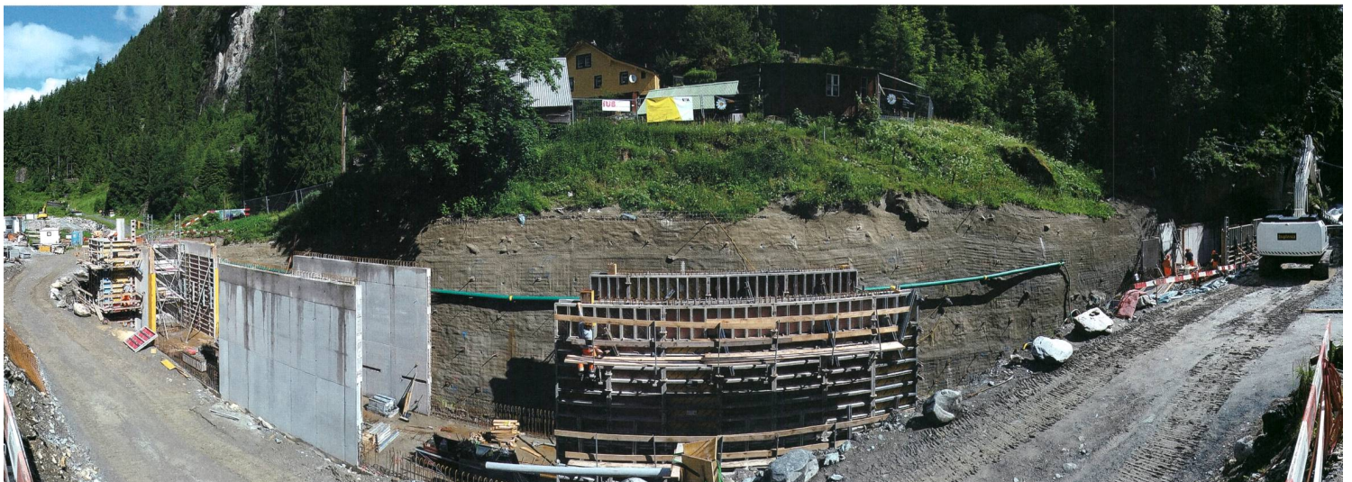
Bild 1 An der Baustelle im Maderanertal sind die Bauarbeiten derzeit in vollem Gang.
