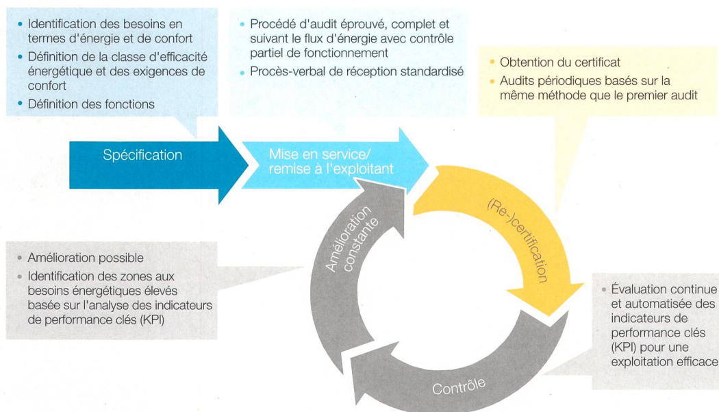
Figure 4 Application du système Eu.bac dans le cycle de vie du bâtiment.
