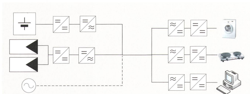
Figure 2 Schéma électrique d'un environnement AC alimenté par le biais du réseau, de modules photovoltaïques et d'un moyen de stockage (à gauche, de bas en haut).
