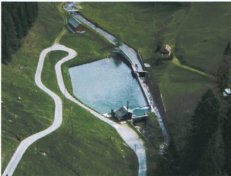
Das Kraftwerk am Niederenbach in Schwanden ist das älteste noch in Betrieb stehende Kraftwerk der kommunalen Elektrizitätswerke. Es wurde am 4. November 1899 mit einer maximalen Leistung von 760 PS eröffnet, mehrmals erweitert und weist heute eine maximale Leistung von 1760 kW auf.
