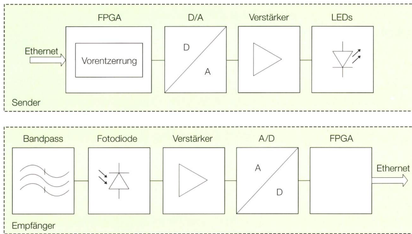
Bild 1 Blockschaltbild Sender (oben) und Empfänger (unten).
