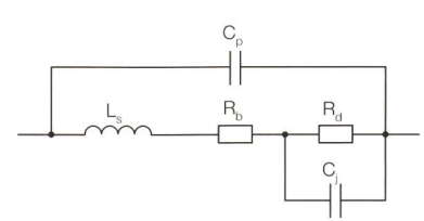
Bild 2 Ersatzschaltung einer LED.
