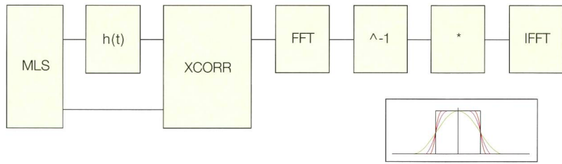
Bild 4 Berechnung der Filterkoeffizienten.
