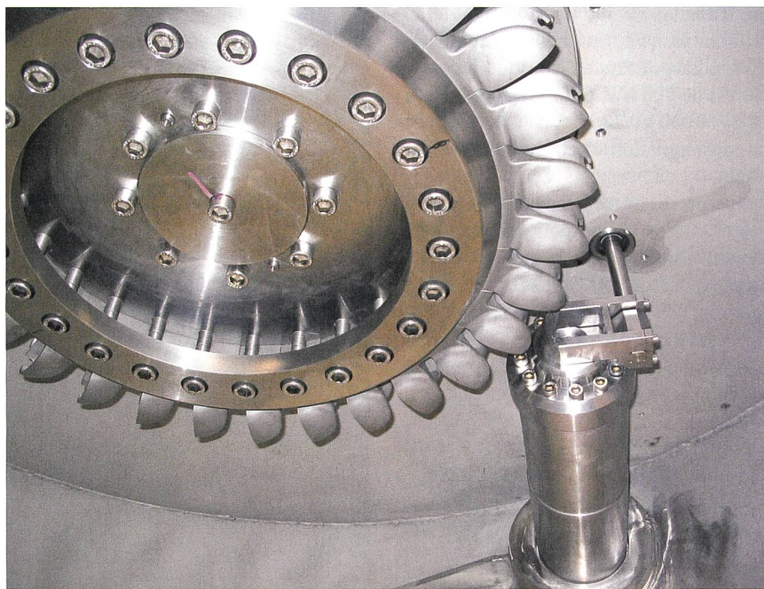
Turbine de Haut-Intyamont FR.
