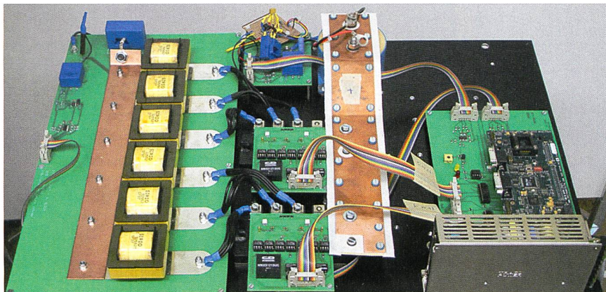
Figure 9 Prototype du convertisseur DC/DC bidirectionnel multibranches.
