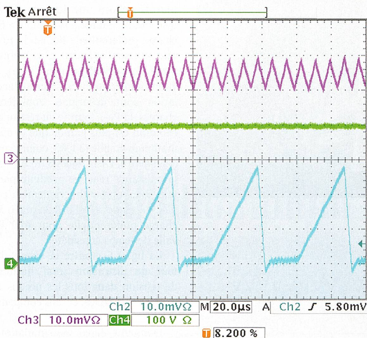
Figure 11 Mesures du convertisseur DC/DC bidirectionnel multibranches.
