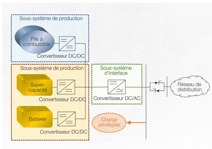
Figure 1 Le système de production décentralisée proposé.
