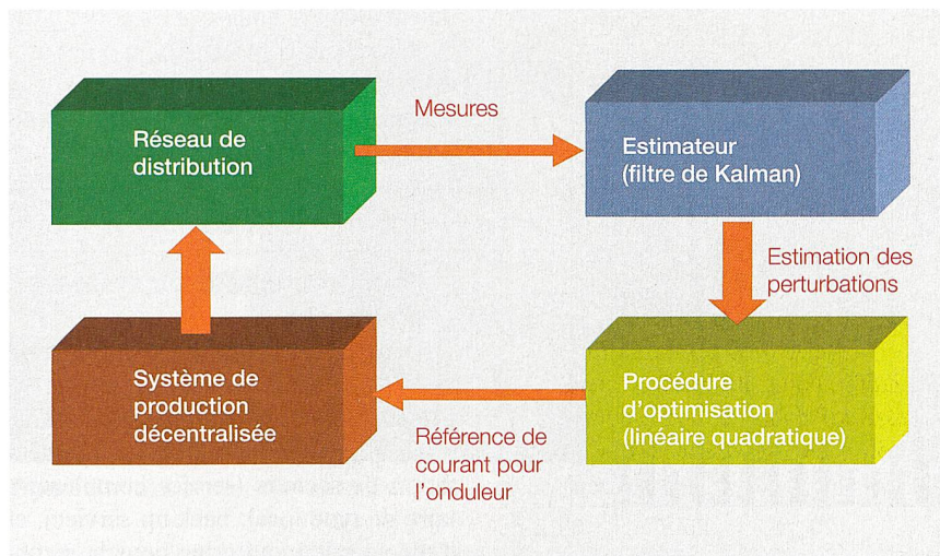
Figure 2 Procédure de génération de références du courant en temps réel.
