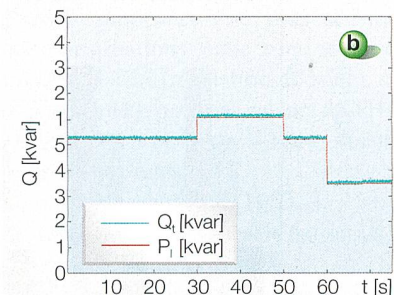
Figure 5 Puissance active (a) et réactive (b) demandées par la charge et fournies par le système de production décentralisée.
