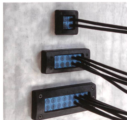
Mehrfacheinführung Roxtec EzEntry von Agro in verschiedenen Grössen.
