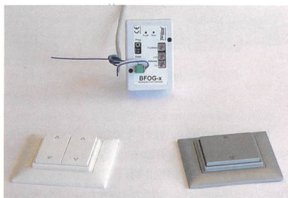
Funktaster und der neue Buskoppler BFOG-x von Wahli erschliessen die für Kabel unerreichbaren Bedienstellen.
