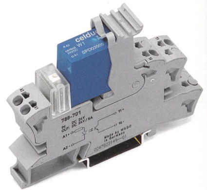
Stecksocket mit Halbleiterrelais aus der Serie 788 der Interface-Bausteine von Wago.
