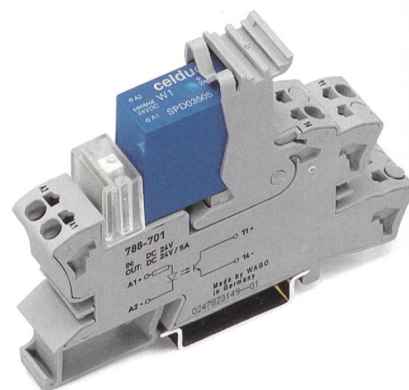
Stecksocket mit Halbleiterrelais aus der Serie 788 der Interface-Bausteine von Wago.
