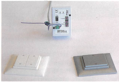
Funktaster und der neue Buskoppler BFOG-x von Wahli erschliessen die für Kabel unerreichbaren Bedienstellen.
