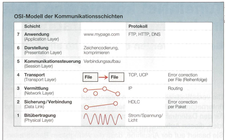
Bild 2 OSI-Schichtenmodell.
