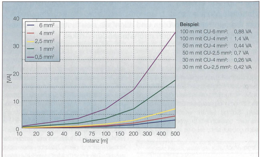
Bild 1 CU-Widerstände – Messleitungen Stromkreise 1 A.
