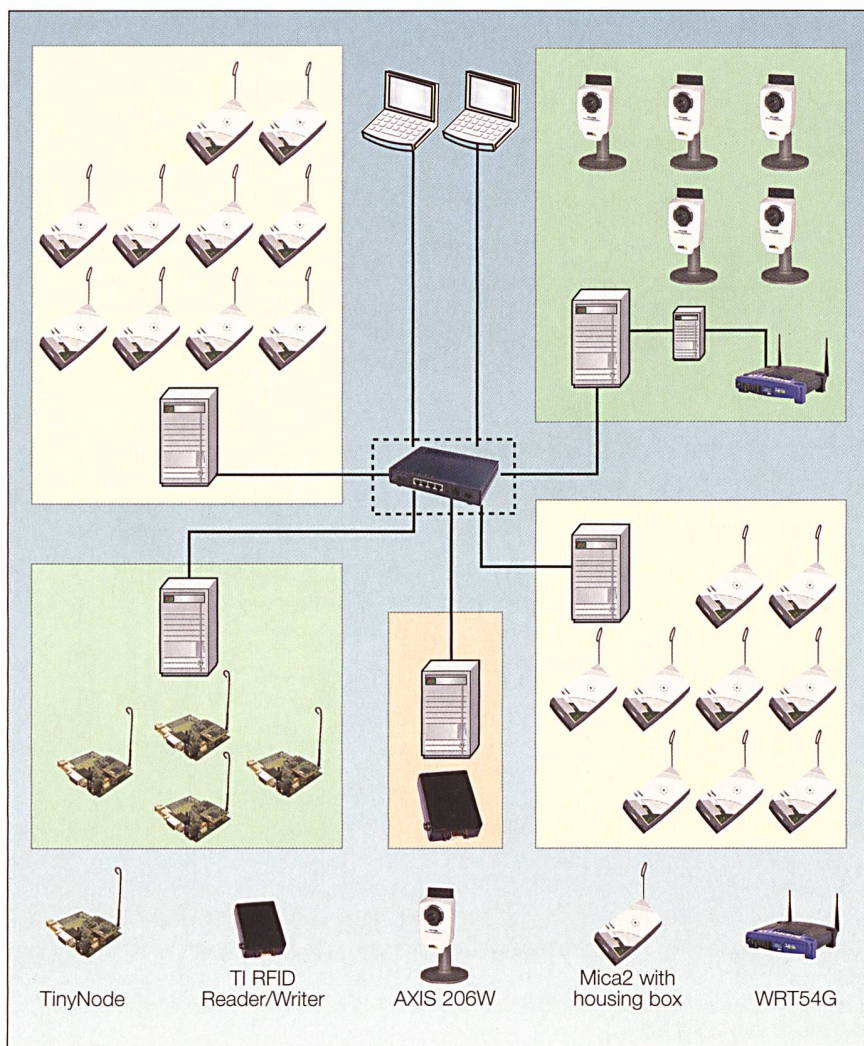
Figure 5 Une configuration des capteurs globaux (GSN) typique.
