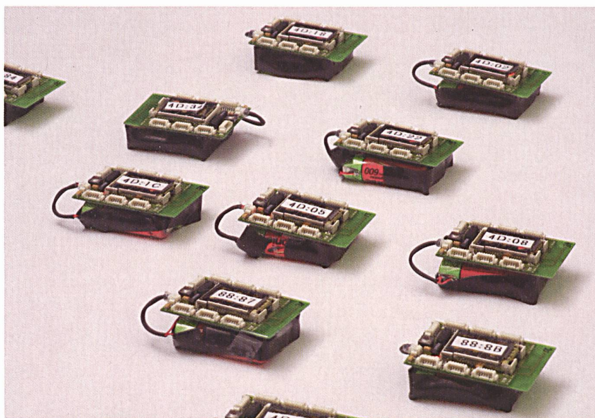
Figure 3 Les BTnodes développés à l'ETHZ.
