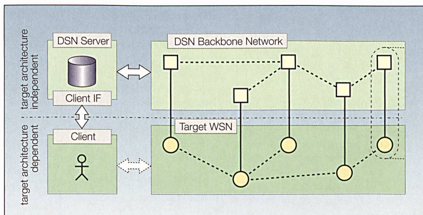
Figure 4 Architecture du réseau de support au déploiement.
