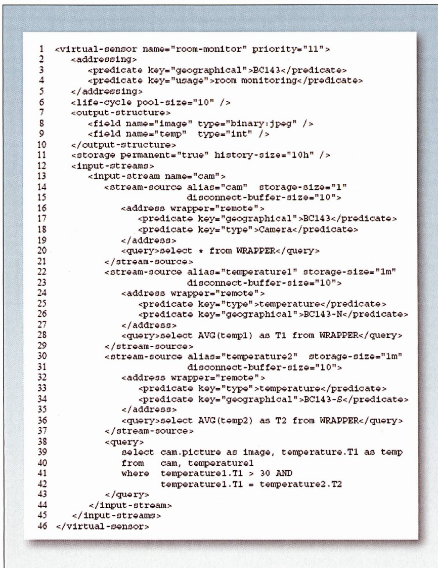
Figure 6 Spécification en XML d'un capteur virtuel.
