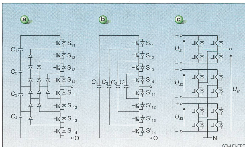
Figure 1 Topologies conventionnelles d'onduleurs multiniveaux
