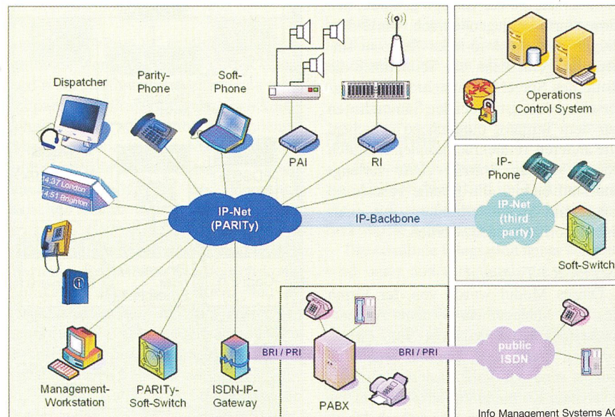
Bild 4 Einbindung verschiedener Endgerätetypen über Internet mittels PA-R-I-Ty
