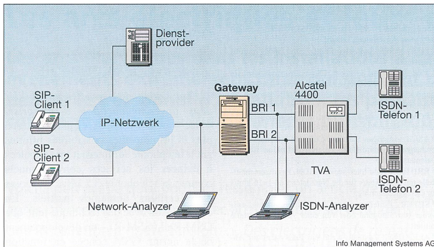
Bild 5 Tests ISDN to SIP
