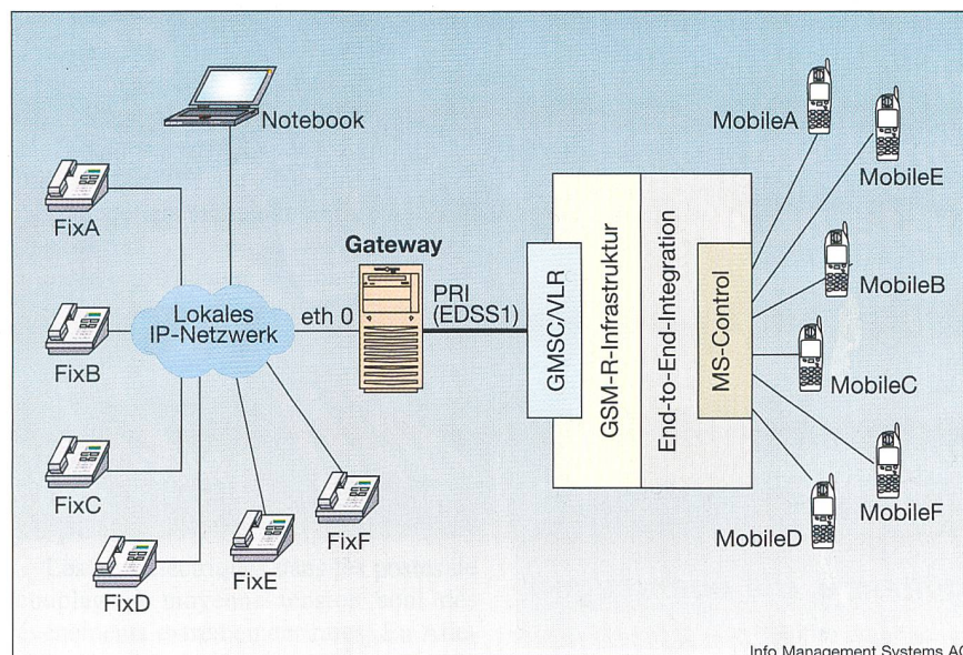
Bild 6 Tests GSM-R to SIP
