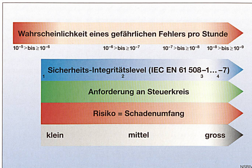
Bild 5 Sicherheits-Integritätslevel nach IEC EN 61508-1...-7
