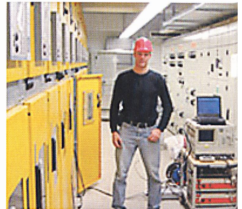
Martin Tiberg misst mit SoFT eine 6,3-Kilovolt-Sammelschiene in einem deutschen Kraftwerk in der Nähe von Düsseldorf.
