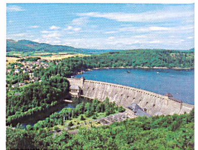
E.ON Wasserkraft will rund 100 Mio. Euro in den Kraftwerksstandort am Edersee investieren. Der Edersee ist mit 27 km Länge einer der grössten Stauseen Europas.
