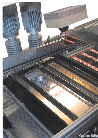
Bild 4 Lokale Stickstoffabdeckung
