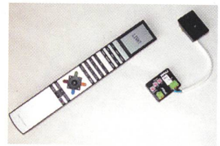
Twiline-Buskoppler «BBO-x» von W. Wahli AG mit Beolink 4
