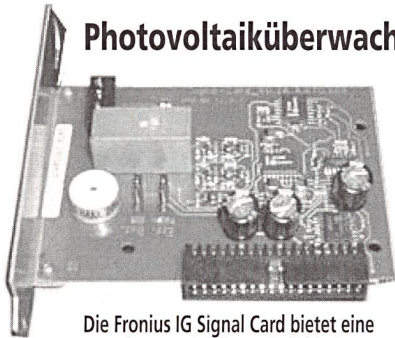
Die Fronius IG Signal Card bietet eine neue kostengünstige Möglichkeit zur Überwachung von Photovoltaikanlagen
