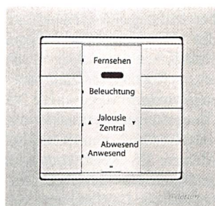
Multifunktions-taster mit IR-Empfänger von Merten:
