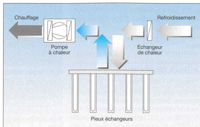
Fig. 3 Vue schématisée du concept de système avec pieux échangeurs
