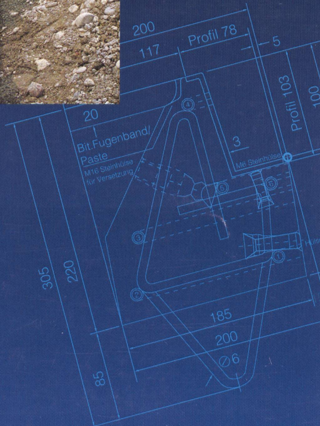
Abdeckungen nivellierbar bis +12 cm
