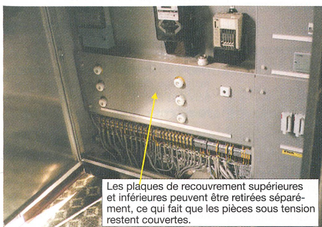
Fig. 8 Plaque de recouvrement partagée: une fois retirée, les pièces sous tension restent recouvertes
