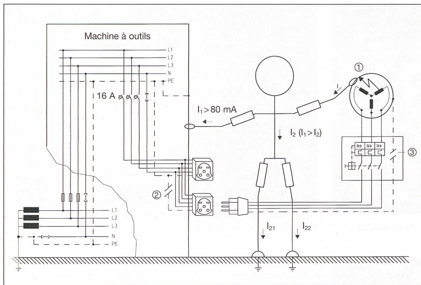
Fig. 9 Pos. 1: court-circuit contre terre de l'enroulement du moteur du convoyeur; pos. 2: interruption du conducteur de protection sur la seconde prise; pos. 3: interruption du conducteur de protection sur le disjoncteur de protection moteur
