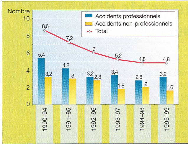
Fig. 1 Nombre total d'accidents professionnels et non-professionnels mortels dus à l'électricité de 1990 à 1999 (moyennes quinquennales)
