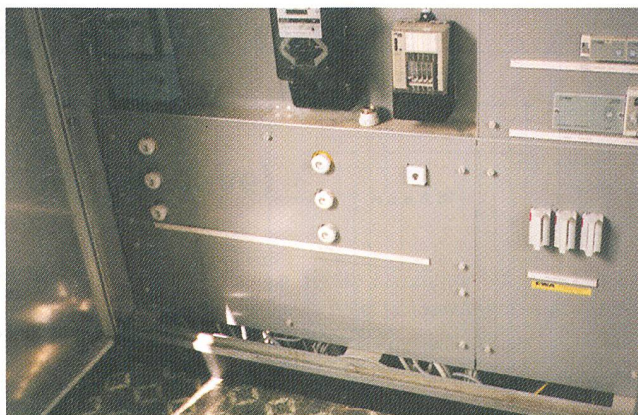
Fig. 7 Plaque de recouvrement non-partagée: une fois retirée, les pièces sous tension ne sont pas recouvertes
