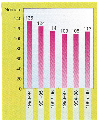
Fig. 2 Nombre total d'accidents professionnels dus à l'électricité des années 1990-1999 (moyennes quinquennales)
