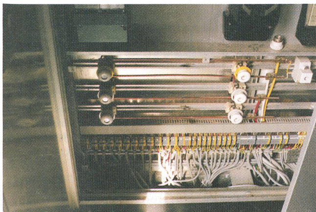
Fig. 6 Recouvrement retiré, bornes et pièces sous tension non-recouvertes
