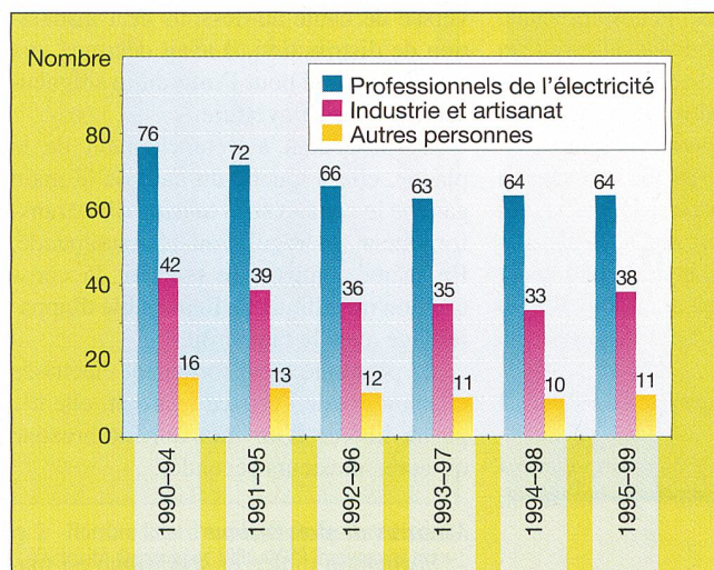
Fig. 5 Nombre d'accidents professionnels dus à l'électricité pour divers groupes de personnes (moyennes quinquennales)
