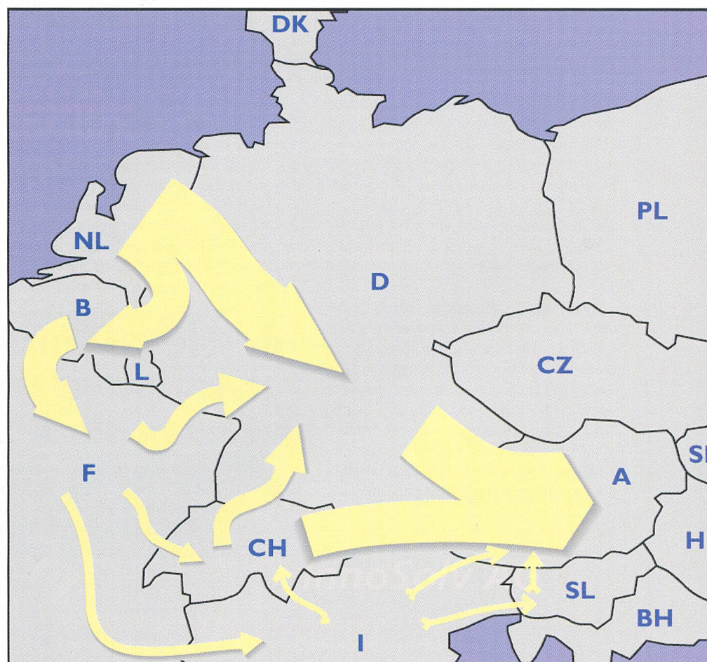
Répartition des puissances dans un réseau interconnecté résultant d'une transaction entre deux partenaires éloignés.
