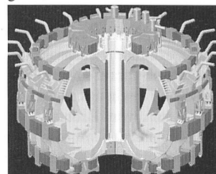
Die supraleitenden Spulen des geplanten Reaktors
