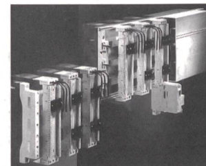
Adaptateurs d'appareils SV multifonctions 25/40 A
